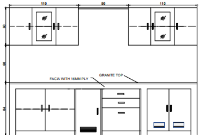
ELEVATION A
