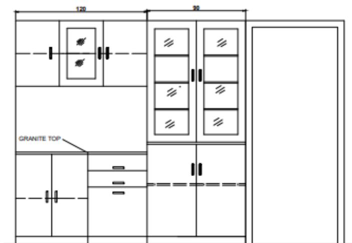
ELEVATION B
